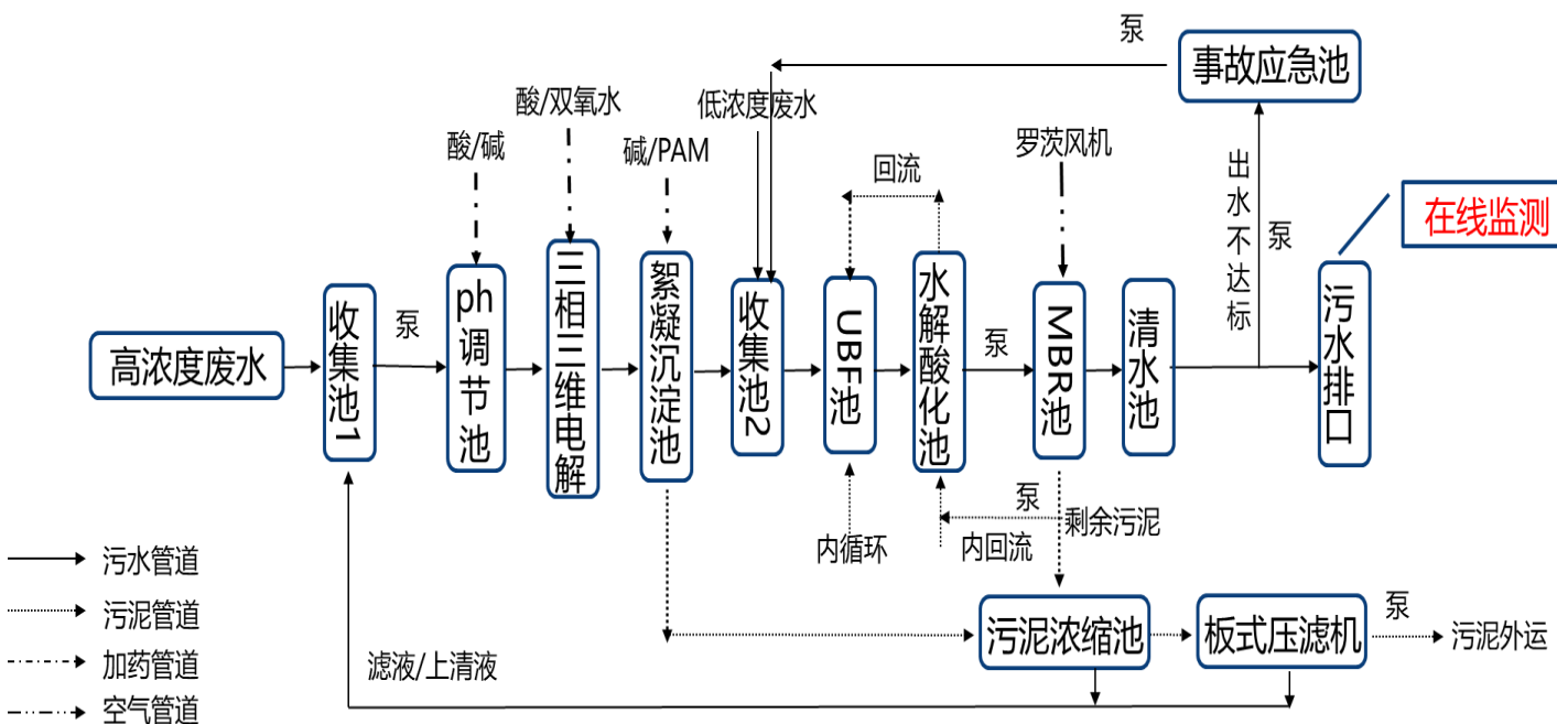
污水站污水处理工艺流程简图
